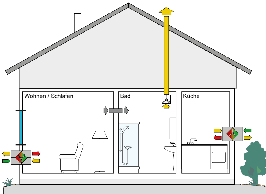
Systemskizze eines Einzelraum- sowie eines Fensterbrüstungsgerätes in einem Einfamilienhaus
