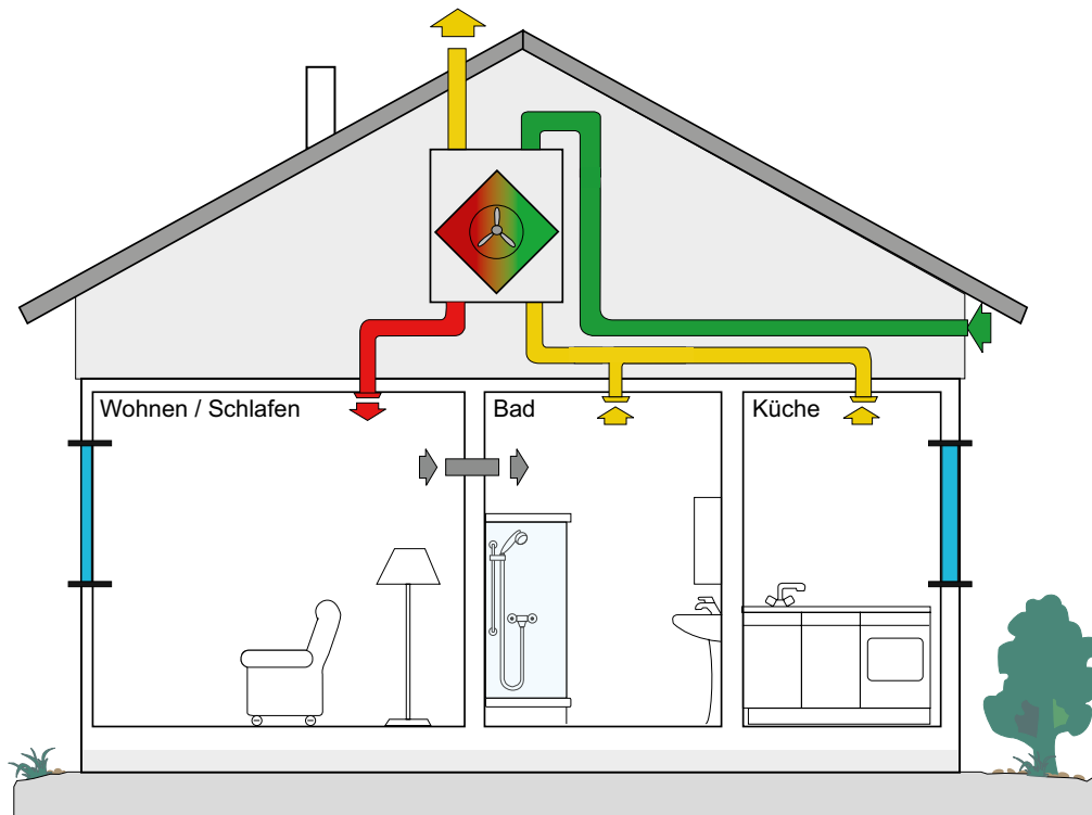
Systemskizze eines zentralen Systems mit Wärmeaustauscher in einem Einfamilienhaus
