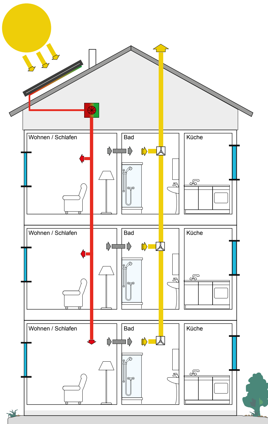
Zu- und Abluftsystem mit solarer Luftvorwärmung in einem Mehrfamilienhaus
