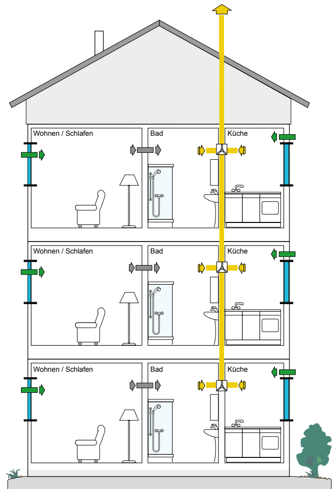
Dezentrale Abluftanlagen mit Zuluftelementen ohne Wärmerückgewinnung in einem Mehrfamilienhaus
